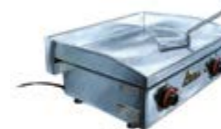
785 Plaque à snacker plancha 220 V / 16A monophasé - 3,3 kW. Ext. : L 60 ; l 40 ; H 19 cm. Température maxi 300°C. Livrée avec 1 tiroir à sauce. 59 Kg
