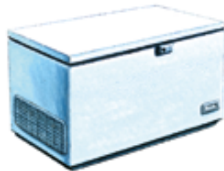
404 Congélateur 600 L 220 V / 16A monophasé - 290 W. Pouvoir de congélation : 30 Kg / 24 h. Ext. L 165 ; P 81 ; H 89 cm. 75 Kg
