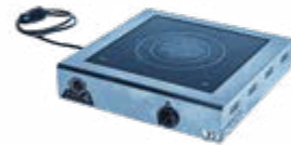
389 Réchaud vitrocéramique 220 V / 16A monophasé - 2,1 kW. Feu Ø 30 cm. 1 bouton de réglage Ext. : L 42 ; l 42 ; H 10 cm. 8 Kg de 50 à 270°C.
