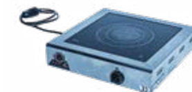
389 Réchaud vitrocéramique 220 V / 16A monophasé - 2,1 kW. Feu Ø 30 cm. 1 bouton de réglage Ext. : L 42 ; l 42 ; H 10 cm. 8 Kg. de 50 à 270°C.
